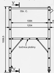
4) Pracovná plošina pre prácu na rovnom teréne
