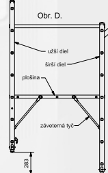
5) Pracovná plošina pre prácu na schodoch
