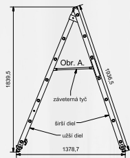
3) Varianta dvojdielny rebrik (štafle) bez opory
