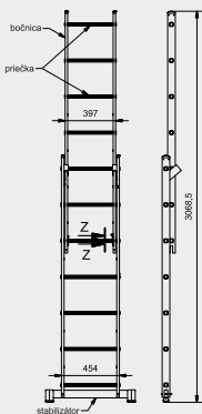
2) Dvojdielny výšuvný rebrik
