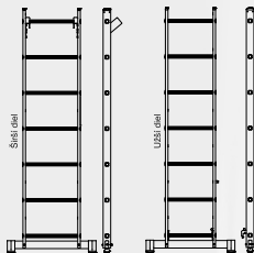
2) Dvojdielny výšuvný rebrik
